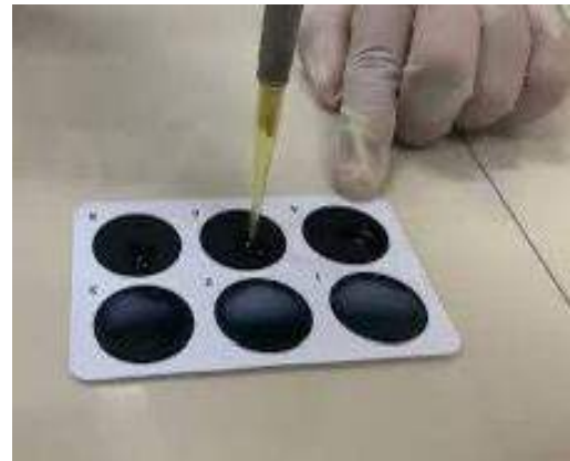
Gambar 4. Pemipetan sampel
