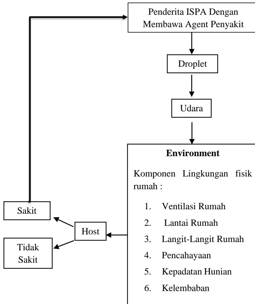
Gambar 2.1 Kerangka Teori
