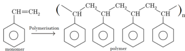
Gambar-1 Polimerisasi Styrofoam (Polistirena) (sumber : Wikimedia)
