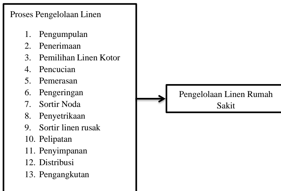
Gambar 2.2 Kerangka Teori
