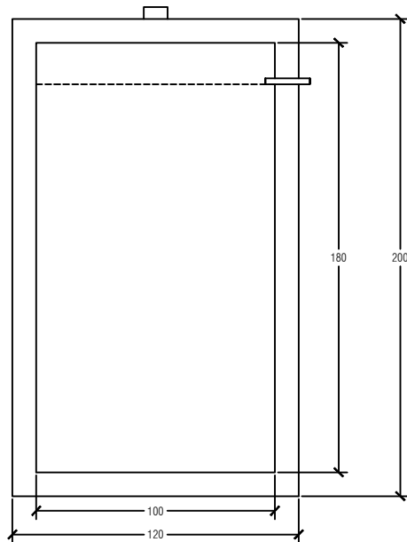
POTONGAN F-F BAK AEROB
