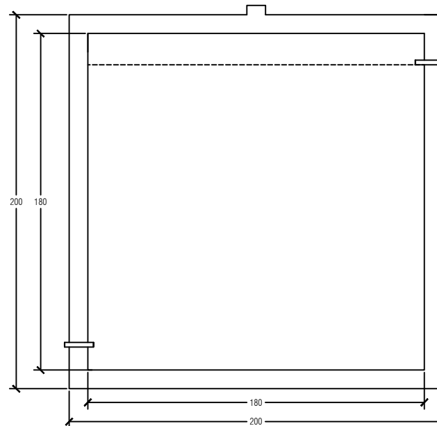
POTONGAN C-C BAK EKUALISASI
